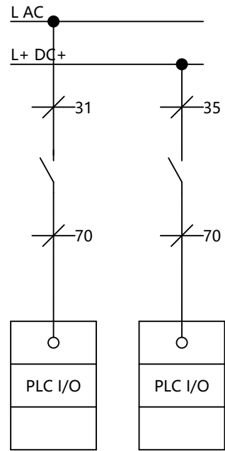
WIRING I/O PLC
